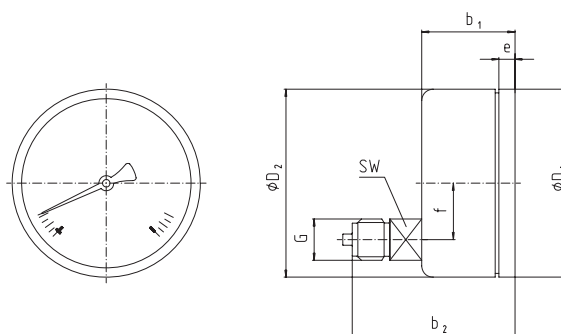
HP 100, эксцентрическое присоединение с тыльной стороны
