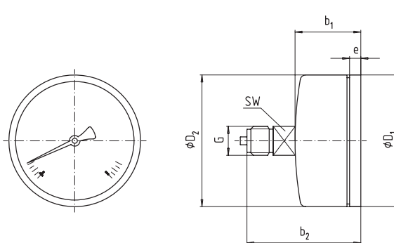
HP 63, центральное присоединение с тыльной стороны
