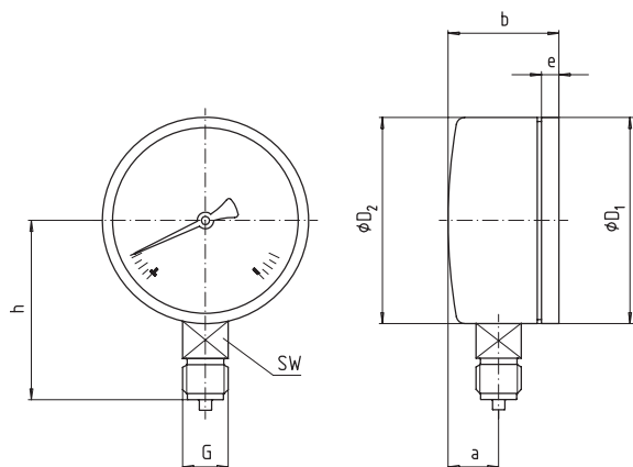
HP 63, радиальное присоединение снизу
